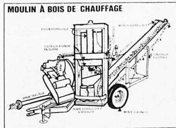
Scie ronde de 30" - Table de 60" - Convoyeur longueur régulière de 12 pieds $30.00 du pied additionnel sur demande Fendeuse Boissée 24" x 24" fend en quatre
