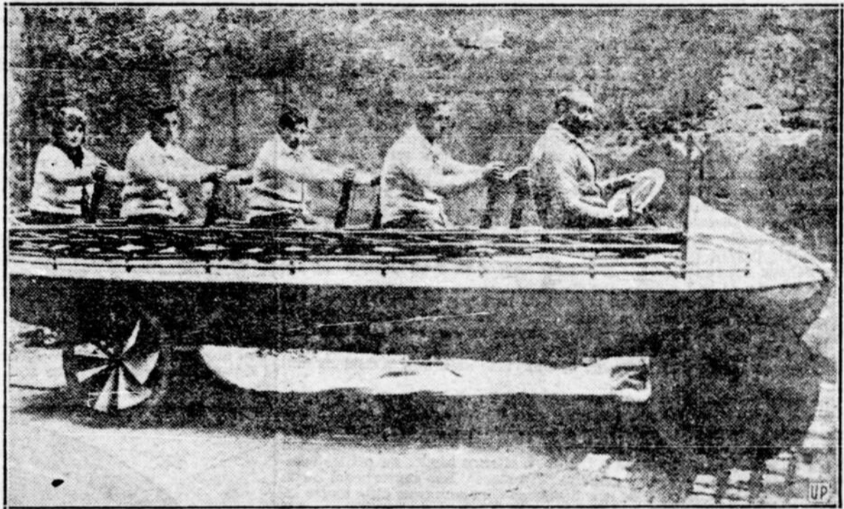
Ou, si vous voulez l'appeler autrement, un "amphibile" fabriqué par un ingénieur allemand pour combiner en un seul tout la chaloupe et l'auto. L'amphibile ou hydromobile marche au moyen de bras ou rames verticales. Une fois dans l'eau la chaloupe avance au moyen d'hélices tournant autour du moyeu des roues de derrière.
