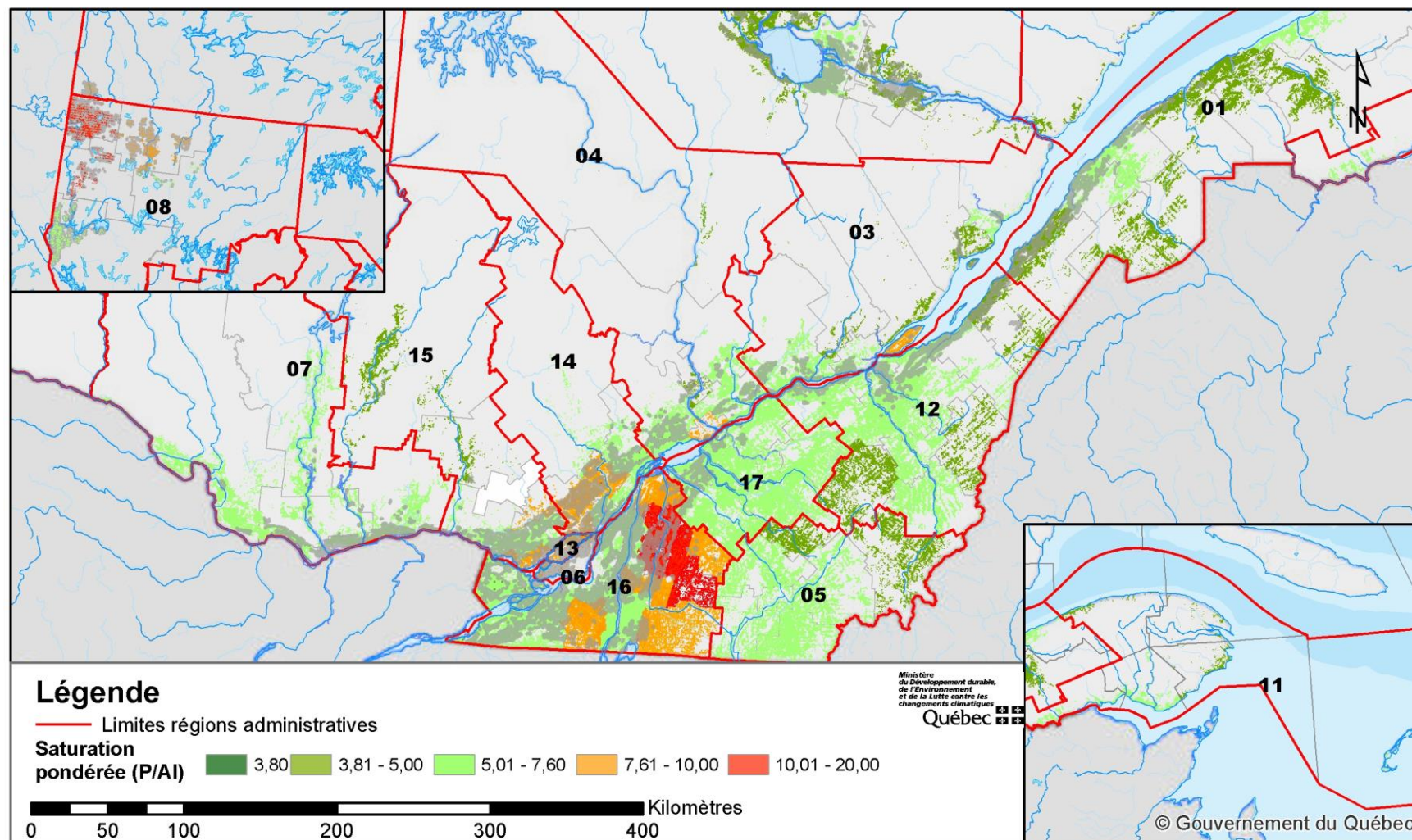
Figure 6. Saturation moyenne pondérée (% P/Al-Mehlich-III) en 2013 en fonction des superficies rapportées dans les classes de saturation (Les données sont corrigées en fonction de l'estimation des superficies « sans analyse »; la partie ombragée correspond aux sols dont la teneur en argile est supérieure à 30 %).
