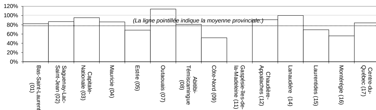
Figure 4. Proportion de la charge de P 2 O 5 contenue dans les matières résiduelles fertilisantes prévue dans les bilans de phosphore et celle réellement appliquée (source : MDDEFP, 2014)
