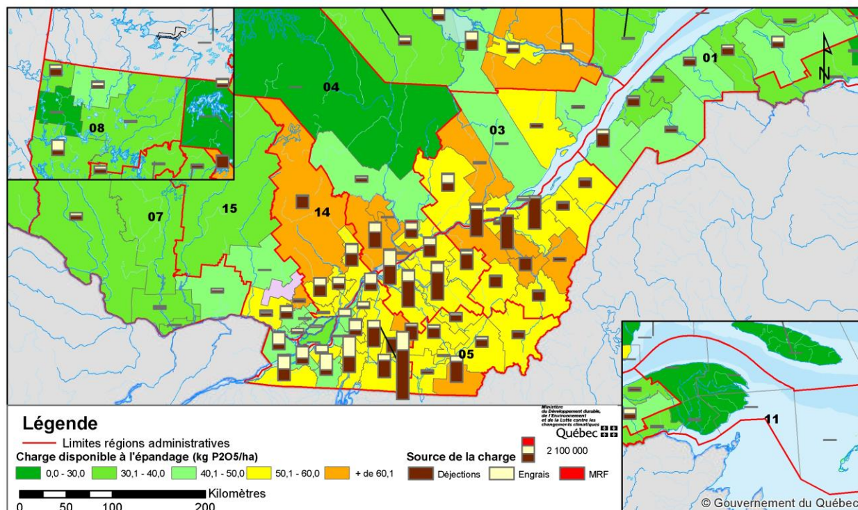
Figure 10. Charge de phosphore disponible à l'épandage en 2013 (kg P 2 O 5 /ha déclaré) et source de la charge de phosphore (kg P 2 O 5 ) par municipalités régionales de comté (MRC)
