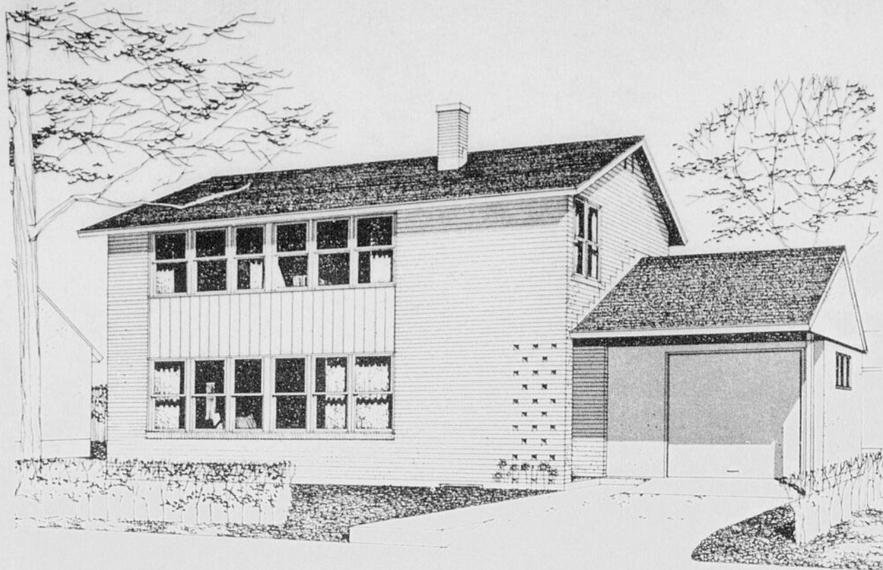
Modèle 514 Architecte: ROY SELLORS, Winnipeg, Man.
