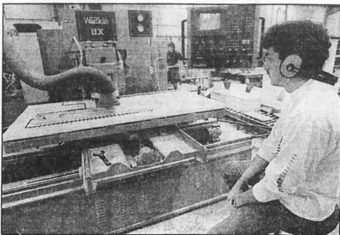
Une «défonceuse» autonome, qui découpe et sculpte le bois en suivant les directives d'un programme informatisé.
