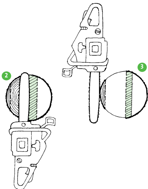
Éclatement du bois (chaise de barbier)
