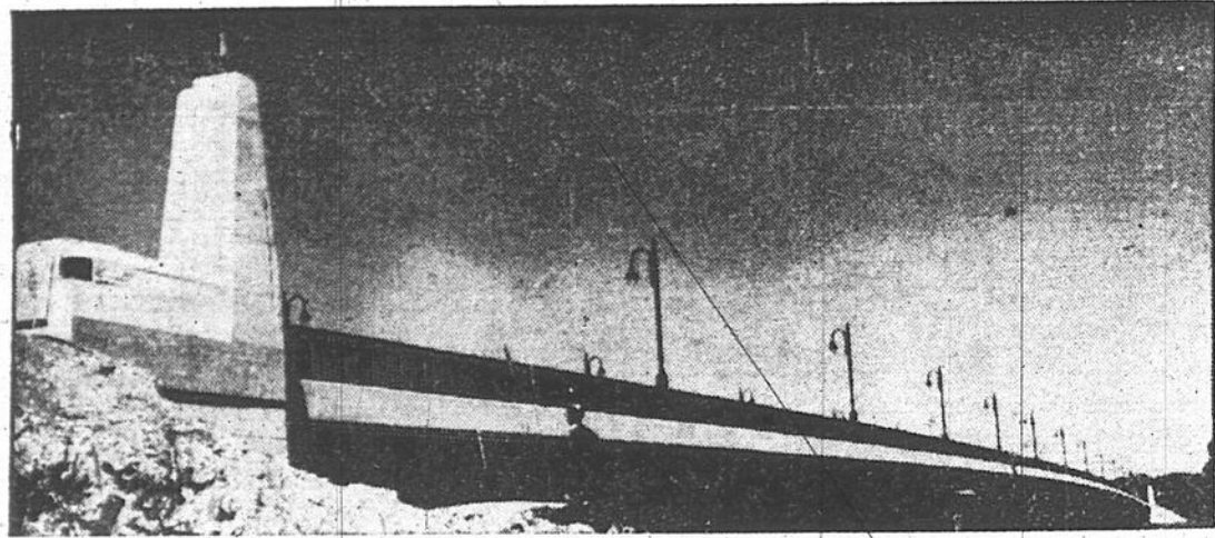
Le nouveau pont Sir Louis-Hippolyte Lafontaine est d'une longueur de 1,548 pieds et d'une largeur de 52 pieds. Une chaussée carrossable de 42 pieds de largeur, bordée de trottoirs de 4 pieds, permet un accès facile et une circulation rapide. Le coût total du pont est d'environ $1 million. Les approches et améliorations de la route ont coûté un demi-million supplémentaire.
