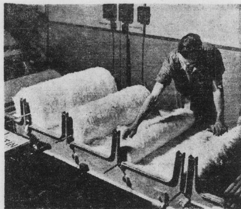
Sur la carte circulaire, on dispose quatre nattes de la peigneuse; elle repeigne et remêle pour constituer un tout plus uniforme et une répartition mieux équilibrée de la laine et du nylon. Le cardage redresse, parallélise, nettoie et fait disparaître les inégalités.
