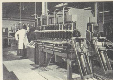
Le ski est mis sous presse.
