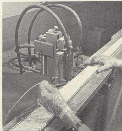
Mise en place semi-automatique des carre d'acier.
