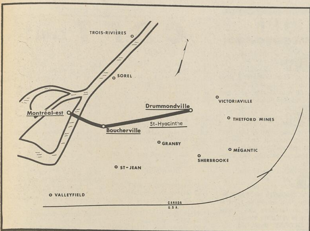
DE MONTREAL A DRUMMONDVILLE -- Ceschemo montre le nouveau pipeline pour la Rive Sud et le territoire qu'il dessert. Ce pipeline de l'Imperial Oil a 60,3 milles de longueur et s'étend de la raffinerie de Montréal-Est jusqu'aux terminaux situés à Boucherville et à Drummondville.
