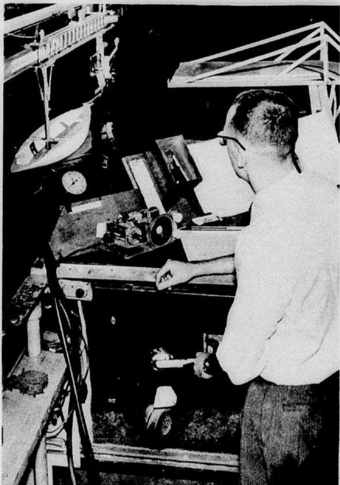
Les modèles de navires passent par toutes sortes d'épreuves à l'Institut de technologie Stevens, à Hoboken, dans le New Jersey. Trois vastes réservoirs sont utilisés ainsi qu'une machine spéciale qui sert à produire des vagues. Les modèles sont fabriqués de bois laminé et à l'échelle. On voit ici un technicien en train de vérifier le comportement d'un modèle de course.
