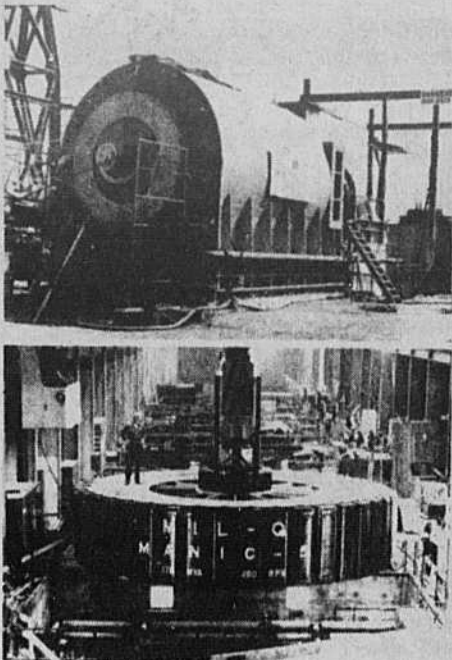
COOPÉRATION TECHNIQUE FRANCO-QUÉBÉCOISE CHEZ MARINE INDUSTRIE DE SOREL. Avec l'aide technique des sociétés françaises Alsthom et Neyrpic, Marine Industrie, de Sorel, construit des turbines, des alternateurs et des compensateurs synchrone de grande puissance. Le ministère des Affaires intergouvernementales du Québec contribue à ce projet en facilitant les échanges de techniciens entre les deux sociétés. Nous voyons (en haut, à gauche) le premier rotor d'alternateur de l'un des huit groupes de 170 MV A que Marine Industrie a construit pour le barrage de Manic 5. La photo du bas nous fait voir la roue Francis, un des 5 groupes de 648 000 H.P., 500 MVA que Marine Industrie construit pour l'usine souterraine de Churchill Falls. Enfin, à droite nous voyons un des quatre compensateurs de 250 MVAR 900 tr-mn, construit à Sorel pour l'Hydro-Québec.
