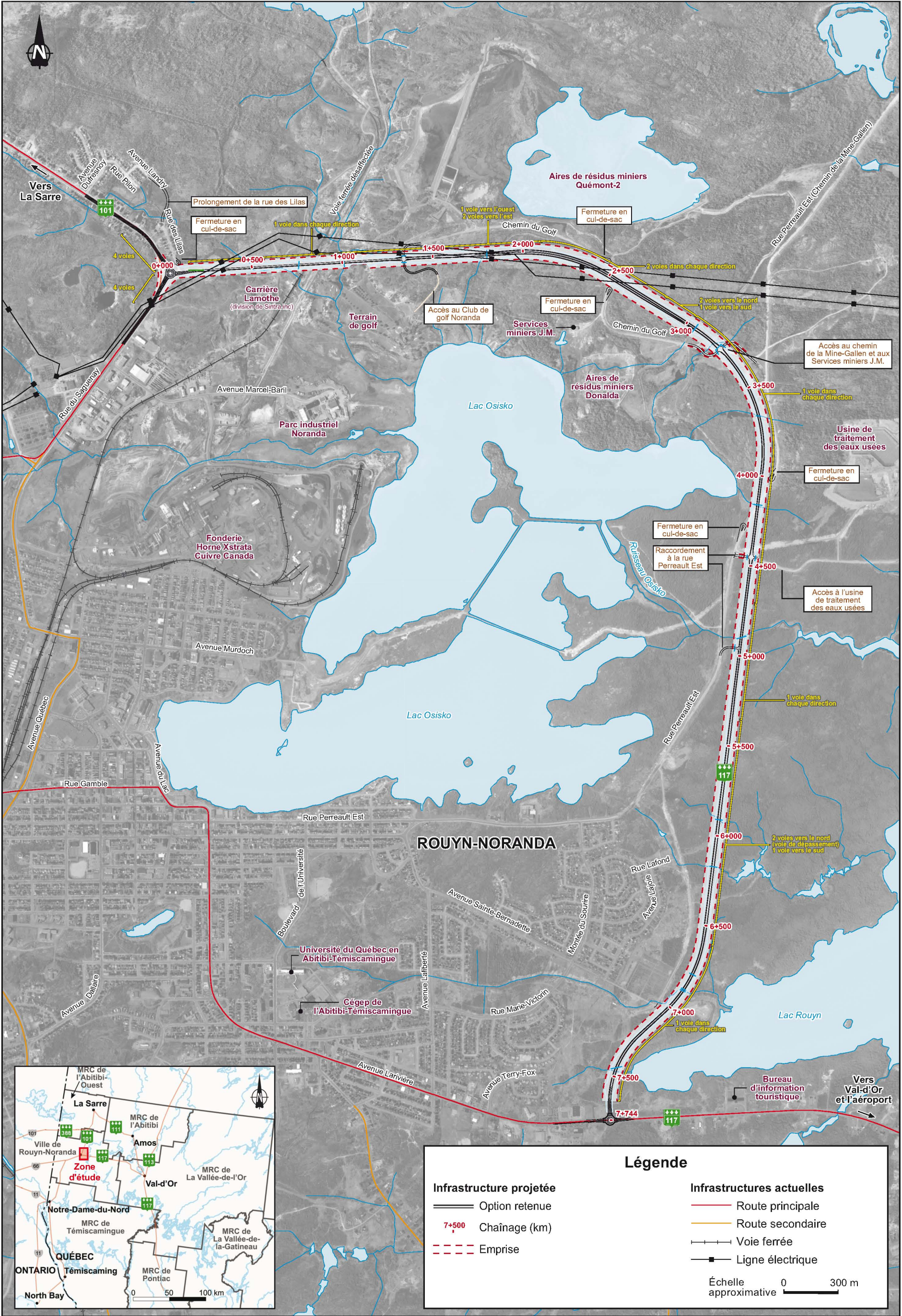
Figure 1 Le projet de construction de la voie de contournement de Rouyn-Noranda, route 117
