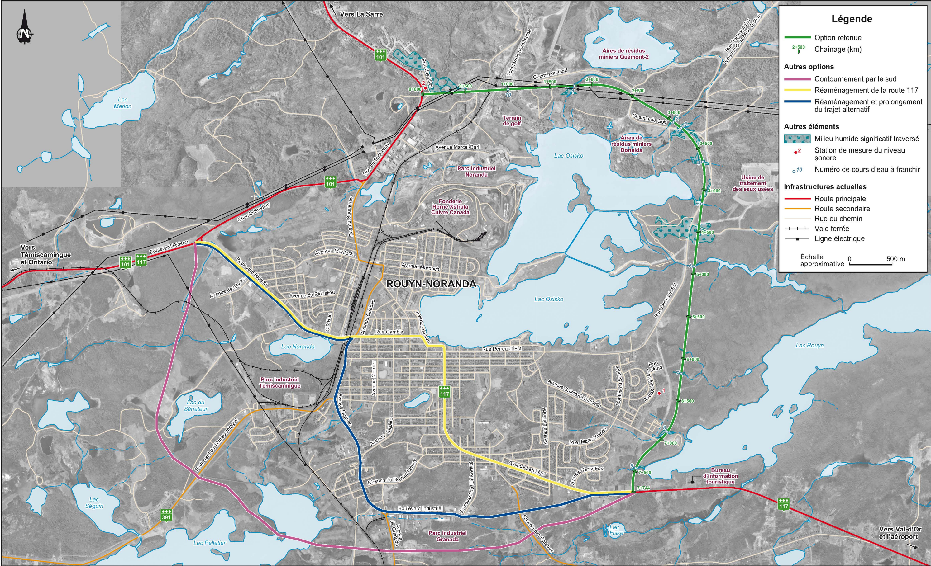
Figure 2 Les variantes de tracés
