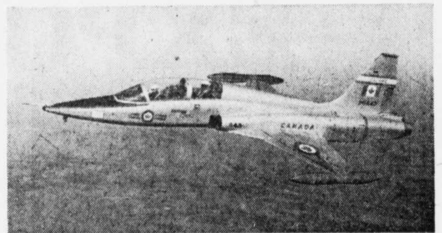
CF 5 — Construit à Montréal par Canadair. Un chasseur utilisé principalement à l'entraînement, il sert également pour la photo aérienne. Le CF 5 peut être monté avec bombes et roquettes dans le cas de support tactique des troupes au sol. Il vole à 1.7 Mach et peut être ravitaillé en plein vol.
