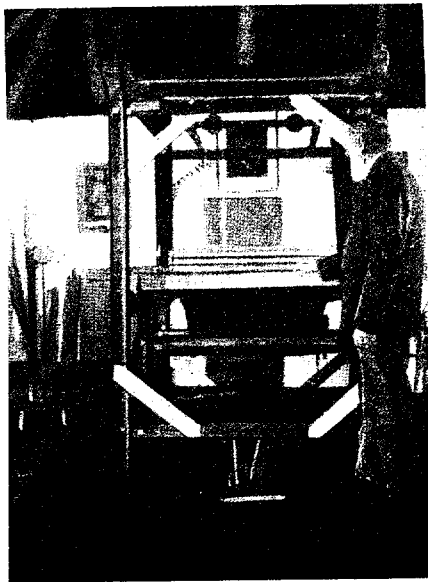
LE MÉTIER CANADIEN CONSTRUIT PAR LE P. LEBŒUF — La première leçon
