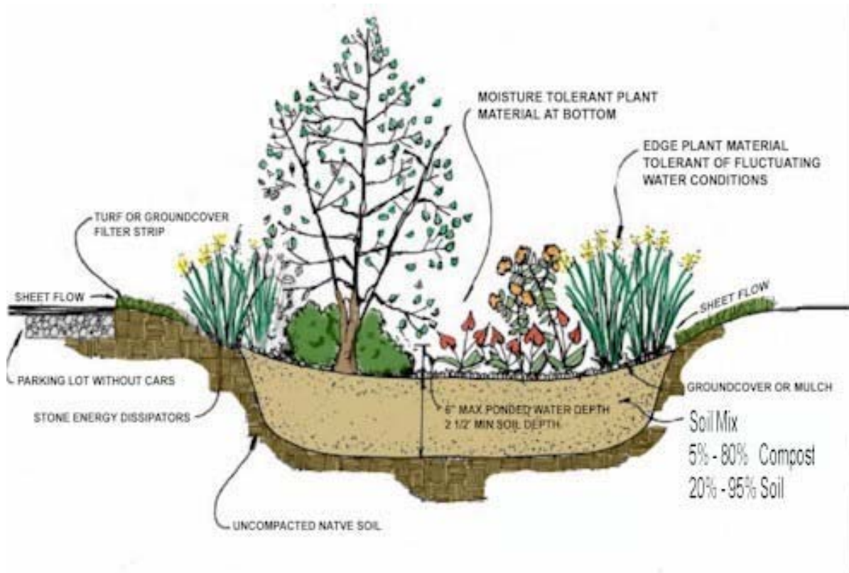
Figure 3.1 Bassin de bio-rétention (tiré de DEP, 2006)
