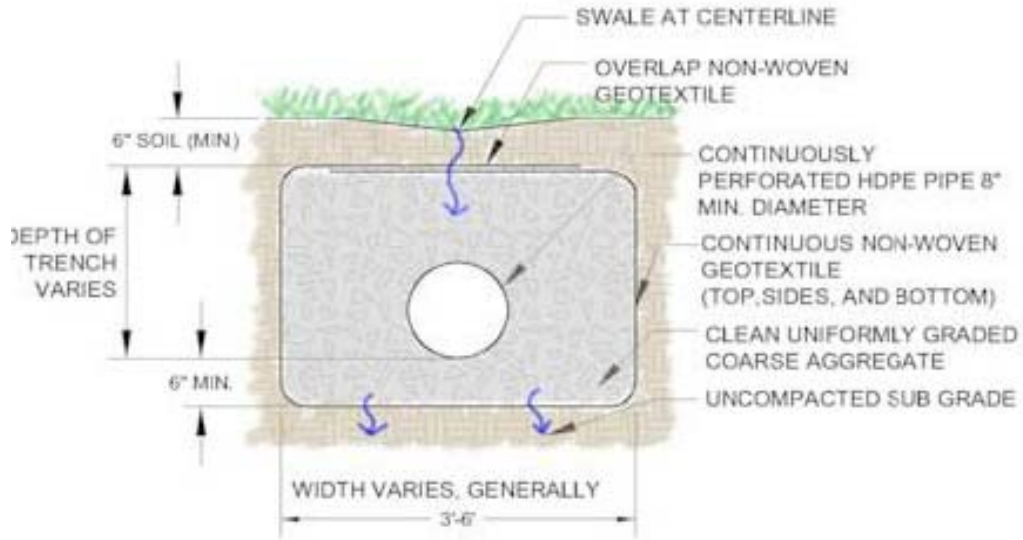
Figure 7.2 Tranchée d'infiltration avec conduites (tiré de DEP, 2006).
