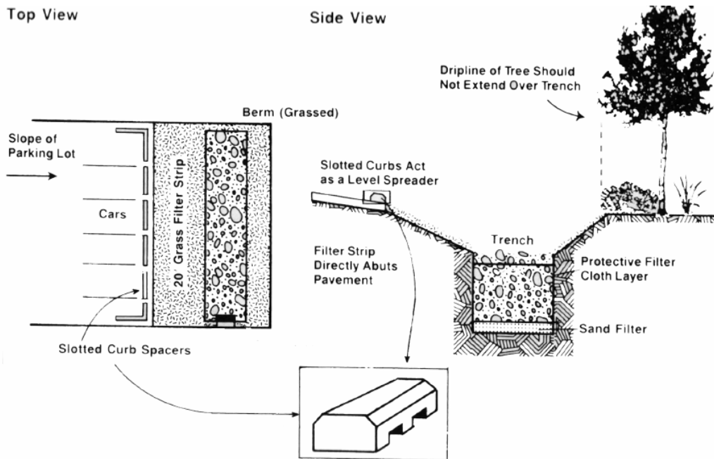
Figure 7.4 Aménagement d'une tranchée d'infiltration en bordure d'un stationnement (tiré de Schueller, 1987).
