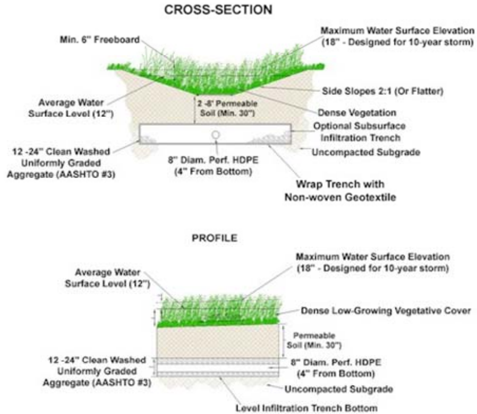
Figure 8.1 Coupes longitudinale et transversale d'une dépression végétalisée (tiré de DEP, 2006).
