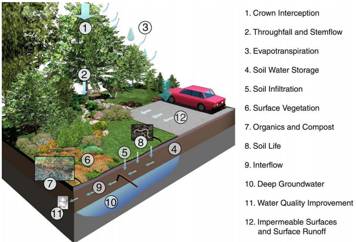
Figure 4.1 Aménagement avec sol absorbant (tiré de GVRD, 2005)
