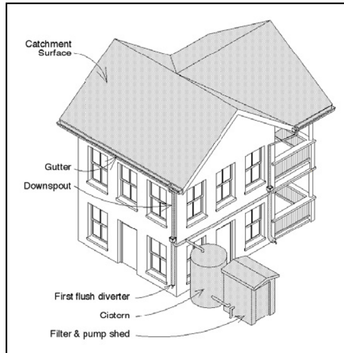
Figure 5.2 Installation typique de collecte des eaux de ruissellement des toits (tiré de TWDB, 2005)
