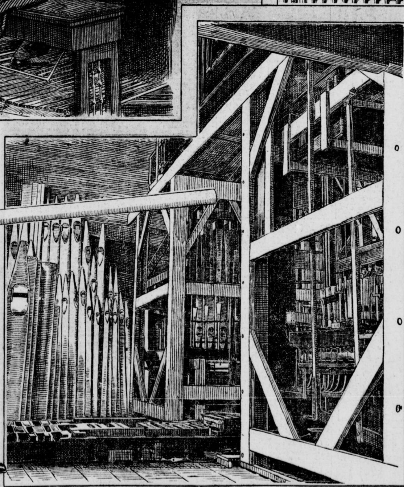
ETAGE DU BAS COMPRENANT LES GROS JEUX DE LA PEDALE ET LAISSANT VOIR VERS LA GAUCHE LA PARTIE HORIZONTALE DU MECANISME.
