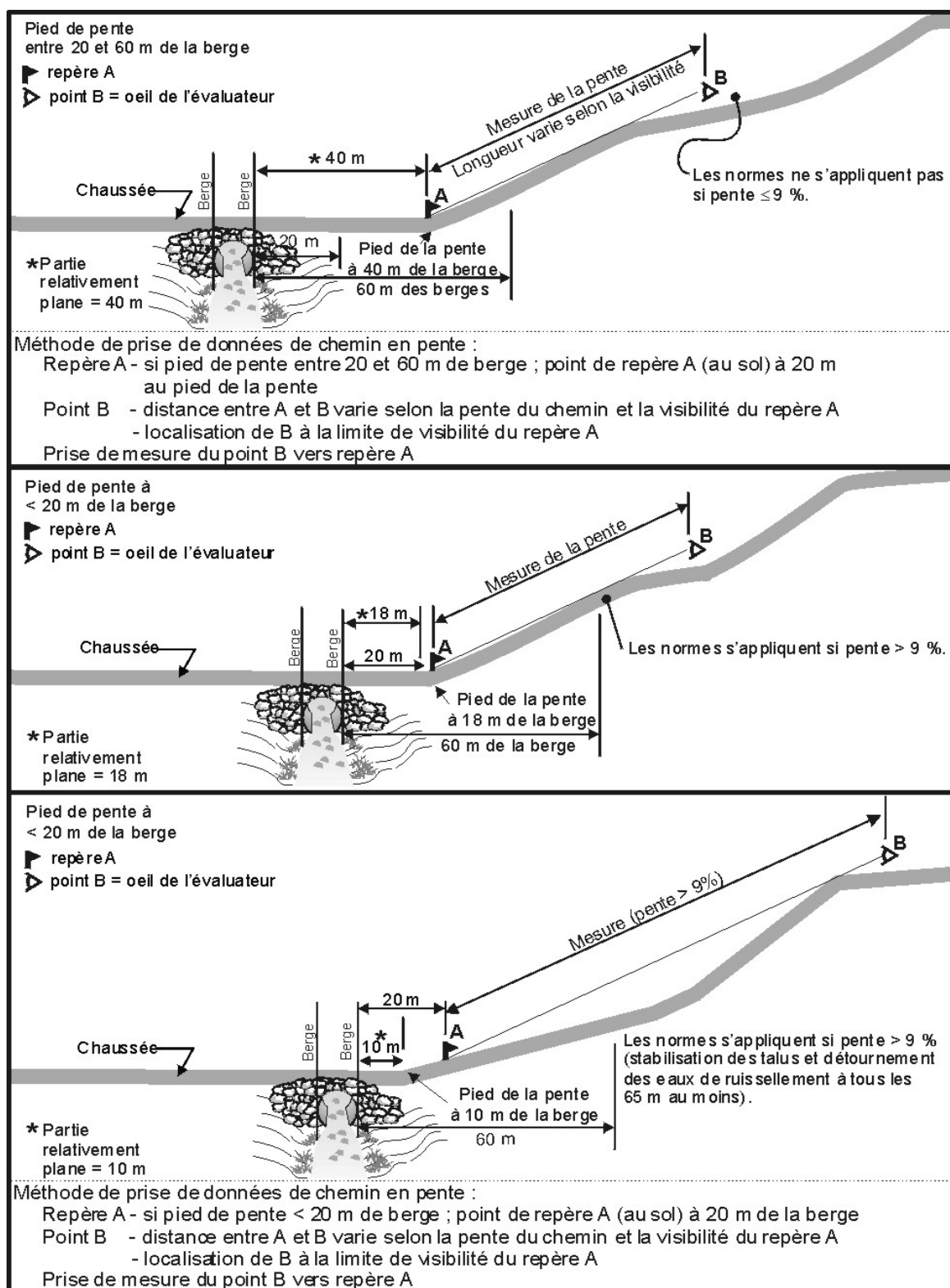
Fig. 2.1.M Méthode de prise de données lorsqu'un chemin a une pente > 9 %.
