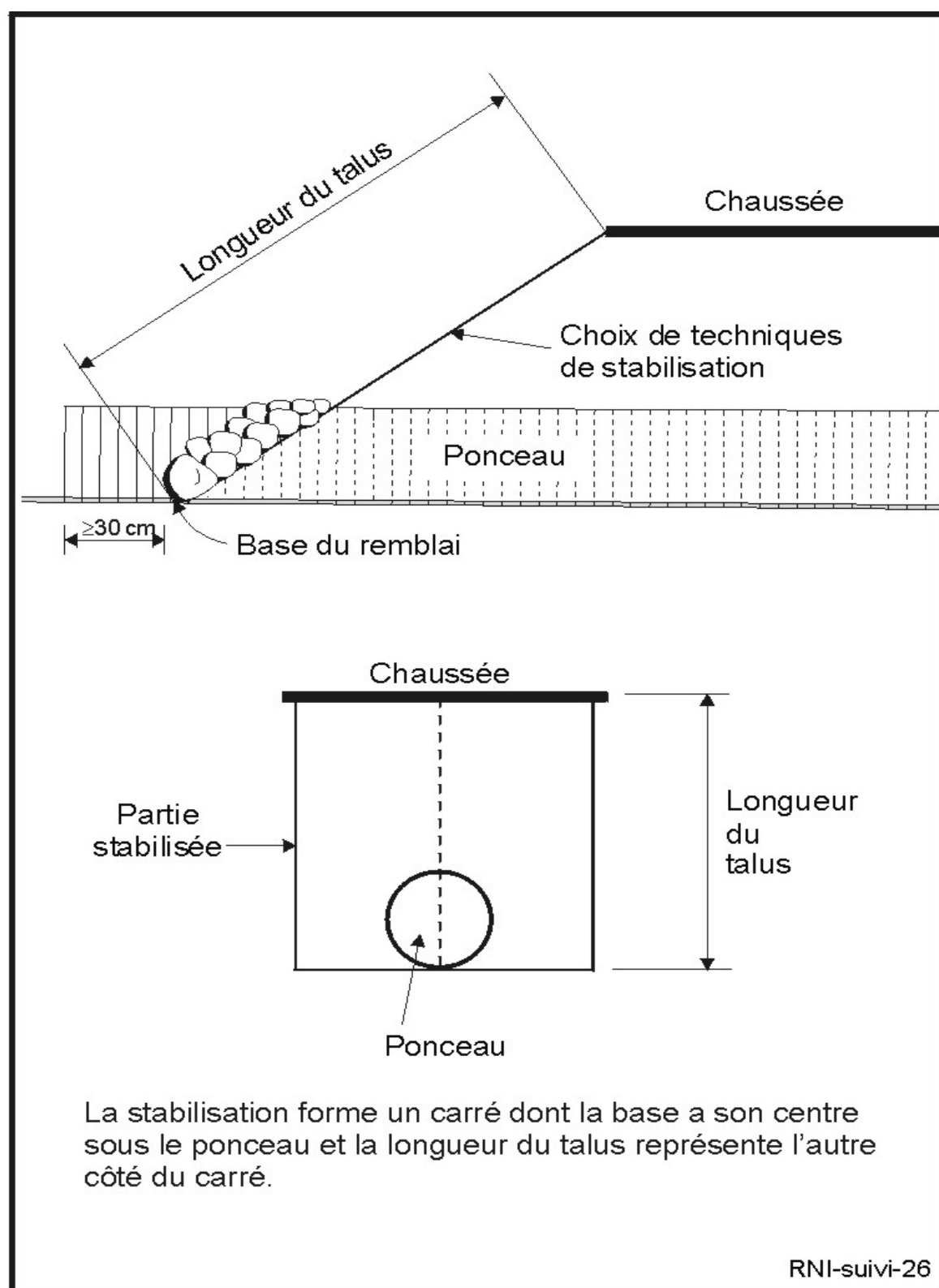
Fig. 4.1.E Stabilisation du remblai autour du ponceau jusqu'à la chaussée.
