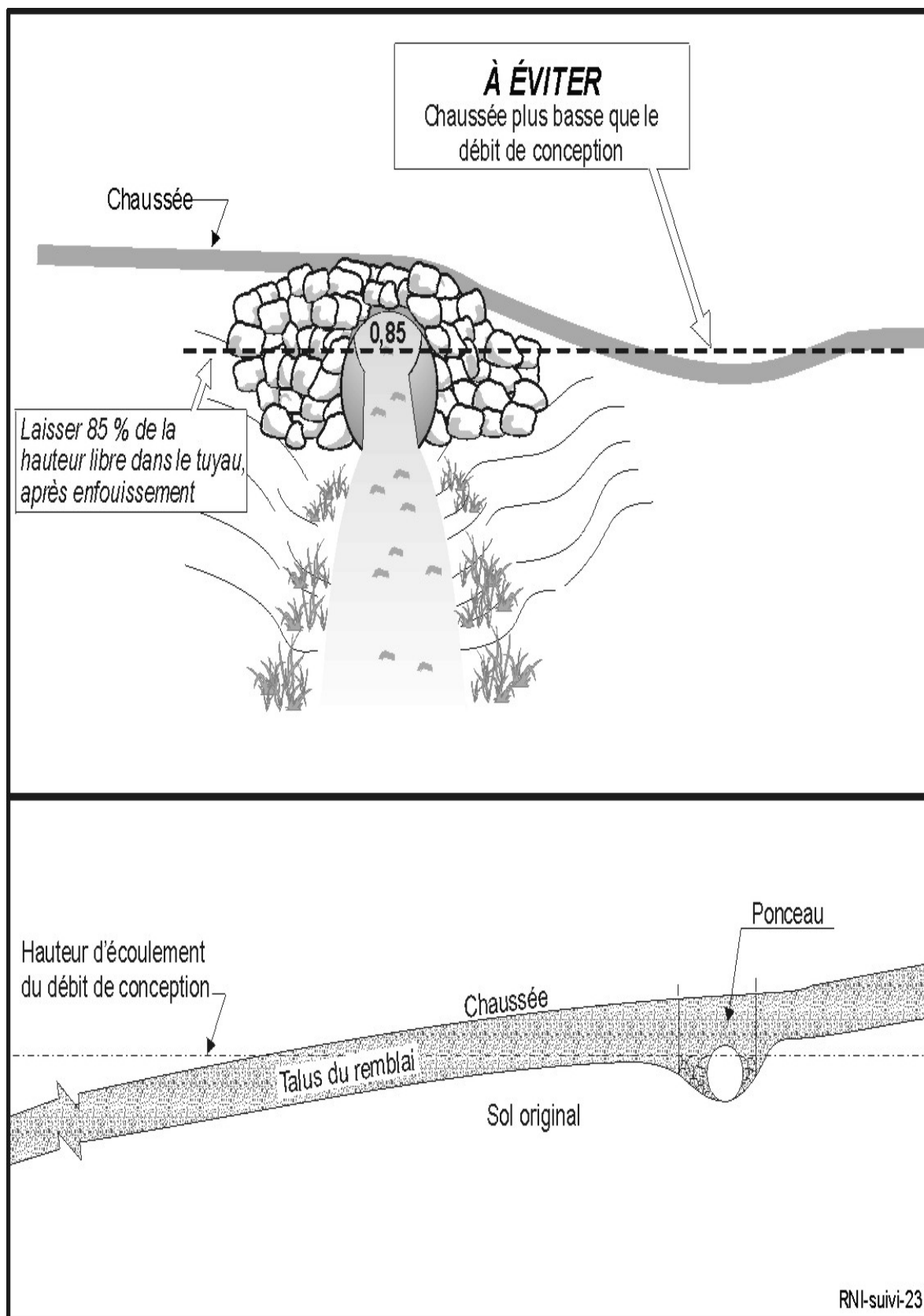
Fig. 2.1.Z. Hauteur de la chaussée par rapport à la hauteur du débit de conception
