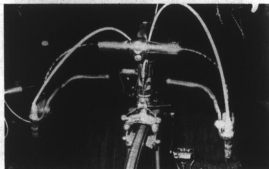
Le guidon recourbé offre trois positions pour les mains. Les freins de la configuration illustrée offrent l'avantage d'être facilement rejoignables quelle que soit la position des mains sur le guidon.
