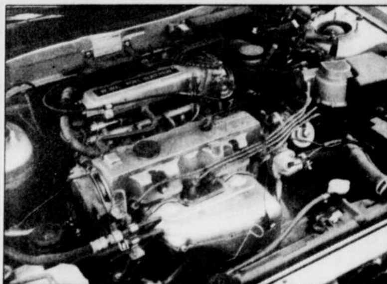
Tout nouveau sous le capot de la 626, le 4 cylindres de 2,2 litres développe 110 chevaux et autorise de bonnes performances. Notons la présence de l'injection électronique et de 3 soupapes par cylindre.
