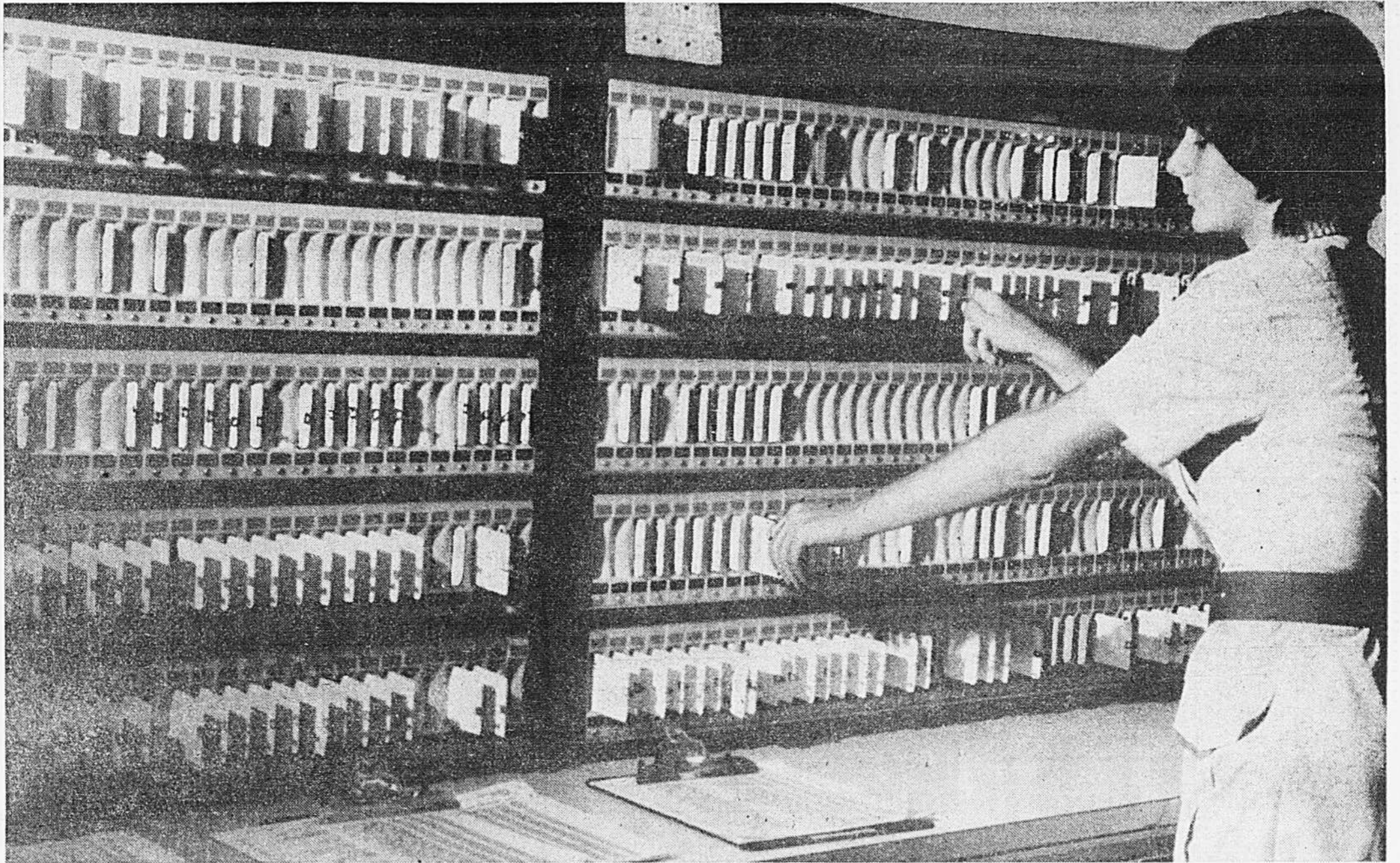
Situé dans le bureau d'enregistrement de l'hôtel, cette console maîtresse est le coeur du système électronique "Cardgard". C'est elle qui contrôle toutes les entrées dans les chambres.
