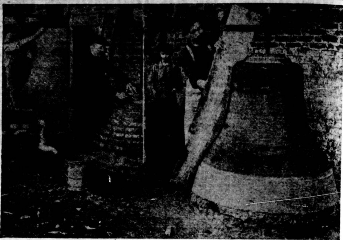
Cette photo, prise dans une fonderie de cloches en France, nous montre les préparatifs de la fonte d'une cloche. Au centre, on aperçoit le moule de briques que l'on revêt ensuite de la fausse cloche (à droite) devant servir de moule à la vraie cloche. Ces deux moules sont recouverts d'un troisième (à gauche) qui laisse un espace libre où sera coulé le métal en fusion. Une fois le bronze introduit dans les moules, on recouvre ceux-ci d'une épaisse couche de terre, afin de permettre le refroidissement lent de la cloche et obtenir une meilleure qualité de son.
