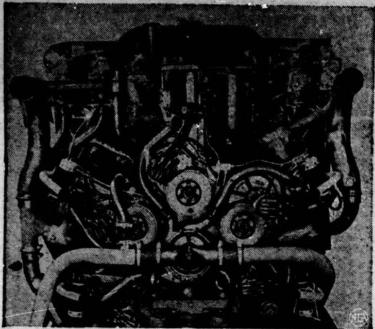
Il est bien à plaindre le mécanicien qui doit découvrir quelque trouble dans un moteur comme celui-ci. Cet ensemble de distributeurs, de tuyaux et de pistons forme le moteur actuel, construit par les usines Chrysler, pour les tanks "General Sherman". Ce moteur est composé de cinq autres engins d'automobile concentrés autour d'un seul arbre de couche.
