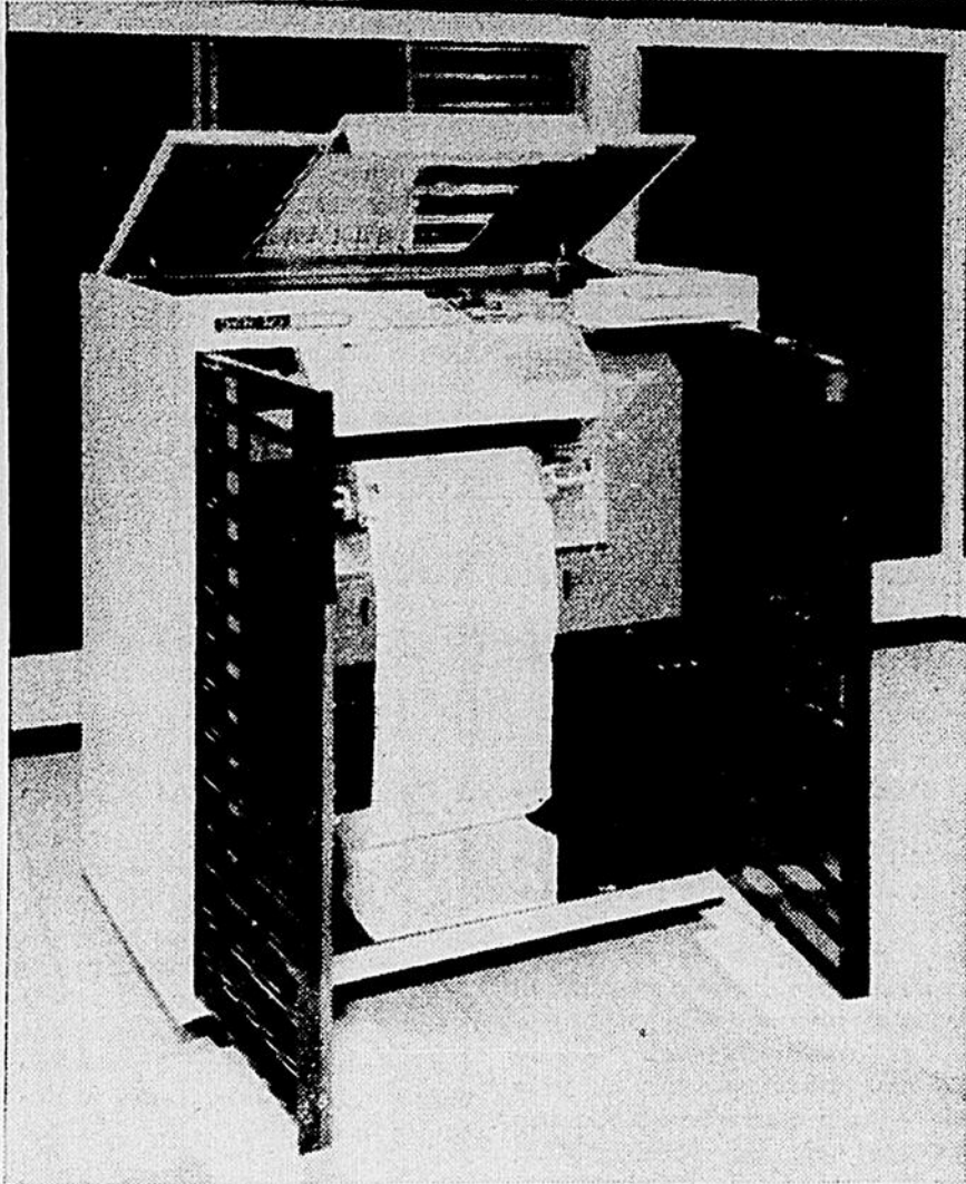
Deux imprimantes rapides de ce type feront partie du matériel du Centre de calcul. Chacune d'entre elles peut imprimer 1,000 lignes à la minute, c'est-à-dire plus de 2,000 symboles par seconde.
