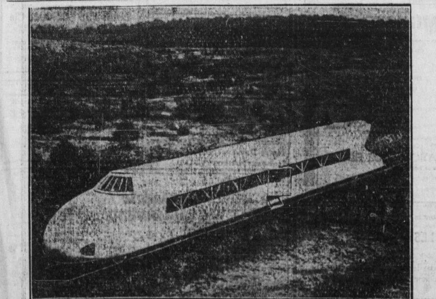
UN WAGON A HELICE — Ce nouveau wagon de chemin de fer, ayant la forme d'un Zeppelin, est actionné par une hélice propulsive. Au cours d'un essai près d'Hanovre, il a fait du 94 milles à l'heure. L'inventeur est Johann Bruckenberg. La voiture a 85 pieds de longueur et est faite en alliage acier-aluminium. Elle pèse 18 tonnes. Cette photographie a été prise pendant les essais.
