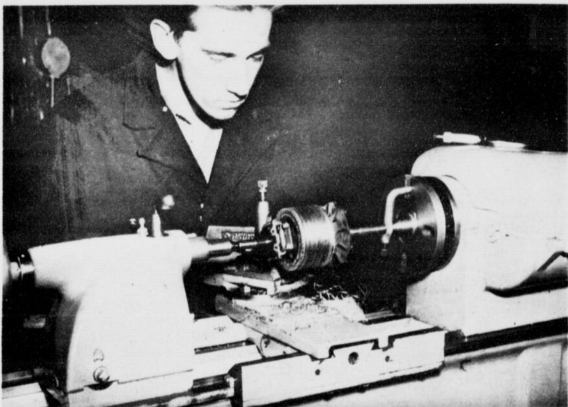
UN AUTRE étudiant surveille ici le travail d'un tour servant à la fabrication d'une pièce de moteur électrique.
