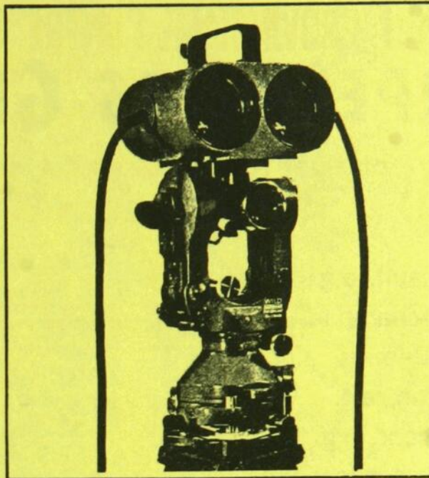
Dispositif de mesures à distance wild Di IOT sur théodolite Universel wild T2
