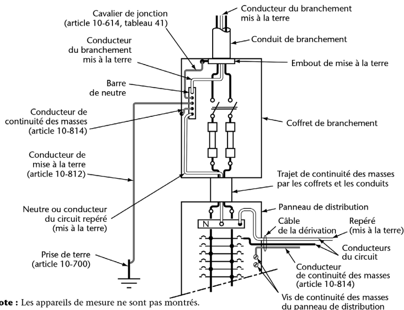
Figure 1 – Conducteurs de continuité des masses et de mise à la terre.
