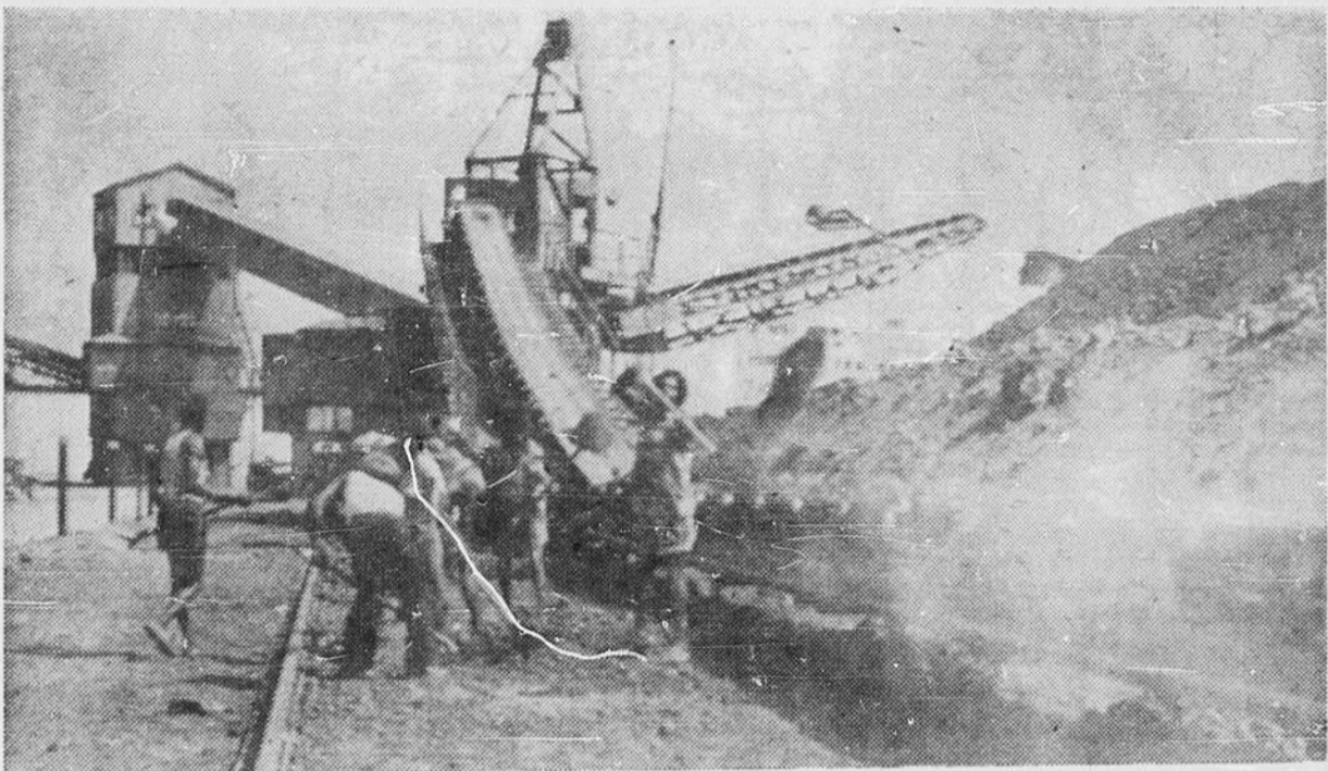
L'installation de chargement de minerai dans le port de commerce de Conakry, en Guinée française.
