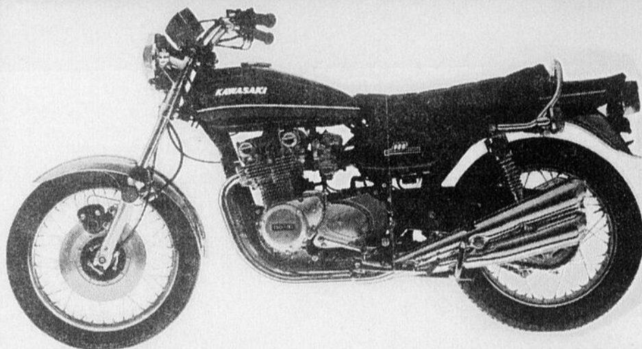
LA KAWASAKI Z1900 est le plus rapide du monde selon la loi; aussi la plus solide. Moteur 2 cannes, 4 cylindres, 4 temps aérés à l'air. 5 vitesses, suspension avant fourche télescopique, amortisseur ajustable.
