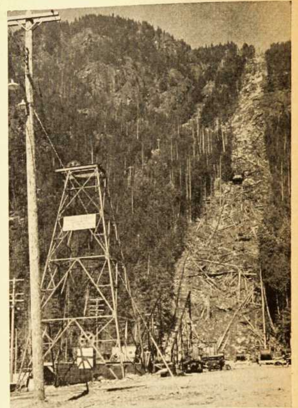
Une trouée a été hâtivement pratiquée dans la forêt pour laisser le passage à un téléphérique qui hisse les ouvriers et leur outillage au sommet du Kemano.
