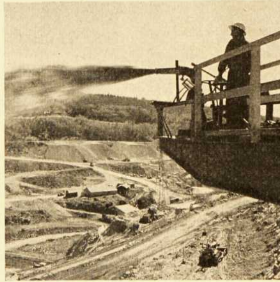
Une vue impressionnante de quelques terrassements effectués à Kitimat. Le matériel de remblai destiné au barrage Kenney, sur la rive Nechako, est arrosé par de puissantes moto-pompes. Ce barrage déviara le lit de la rivière vers l'Ouest et retiendra un vaste plan d'eau.
