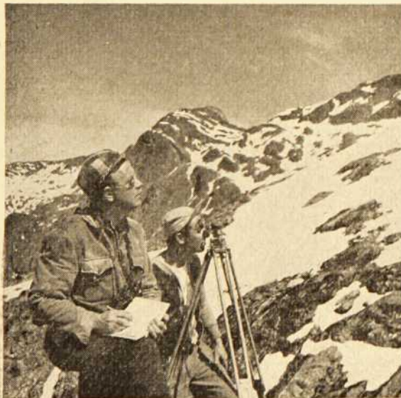
Des ingénieurs-géomètres transformés en alpinistes tracent la route que suivra la ligne de transmission sur le col Kildala, soit à plus de 5,000 pieds.
