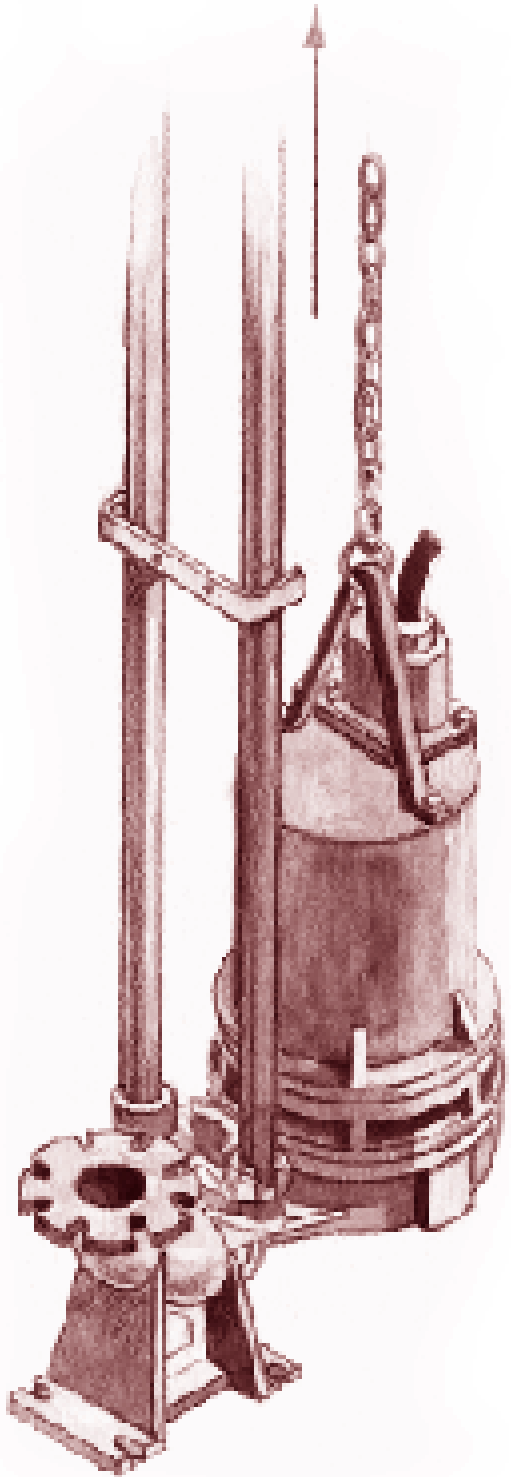
Figure 8 Pompe submersible à coulisseau
