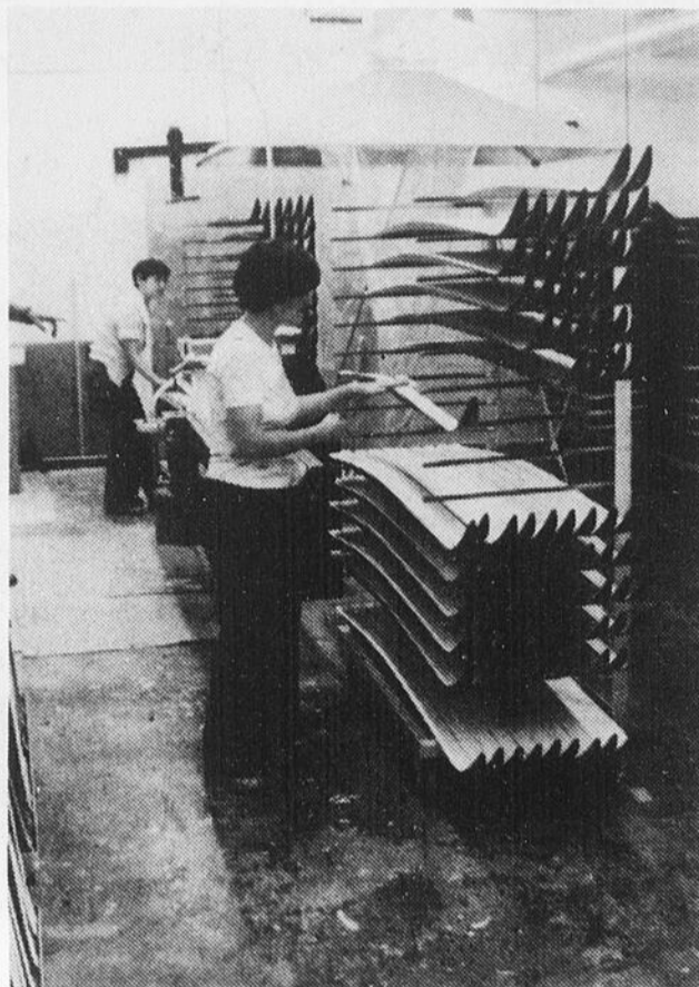
On approche du produit fini, déjà le ski pourrait être utilisé. Il ne reste plus qu'à y donner les couleurs qui en feront définitivement un ski de première qualité signé Karhu-Pinso Canada. [adion]
