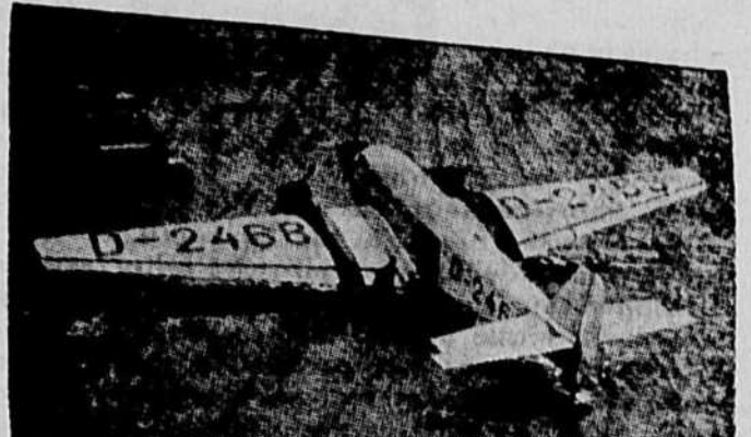
Fig. 1 - D. R. Draco, machine employée pour les services anglais et australiens. Quatre moteurs de 205 chevaux. Peut transporter 2,400 livres. Vitesse maximum: 170 milles à l'heure.
