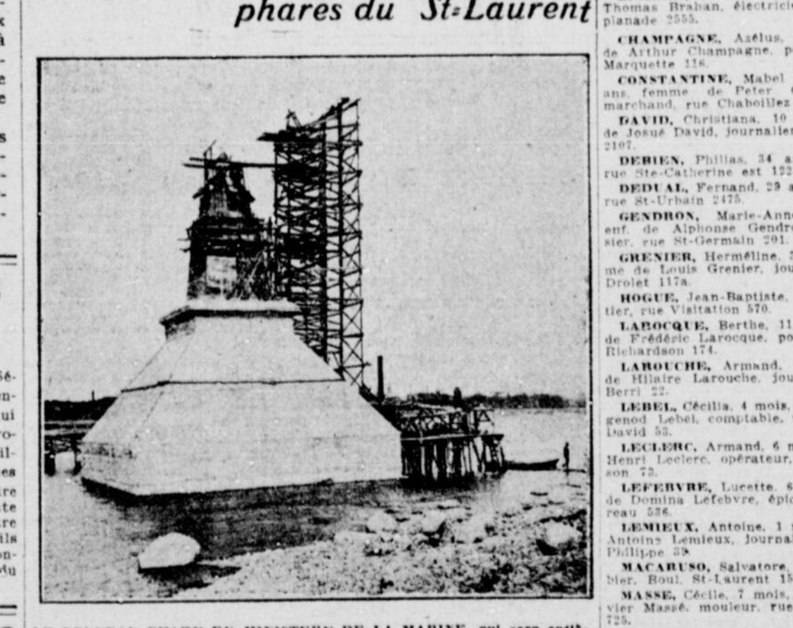
LE NOUVEAU PHARE DU MINISTÈRE DE LA MARINE, qui sera entièrement terminé vers le 7 août. Ce sera le plus puissant des phares du district de Montréal. La base est faite de béton armé et capable de résister à tous les efforts des houles de glace. Sa hauteur est de 87 pieds et sa base avec la tour proprement dite a 47 pieds. La tour a 47 pieds de tour et sa lumière aura un diamètre de 3 pieds 6 pouces et pourra lancer des jets de lumière à une distance de 7 milles. Un escalier de fer conduit à la tour.
