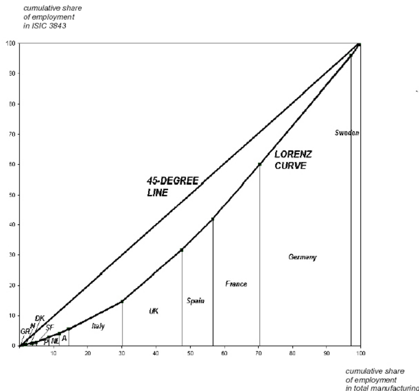
Figure 5.2 Courbe de Lorenz (concentration filière « Véhicules moteurs »)
