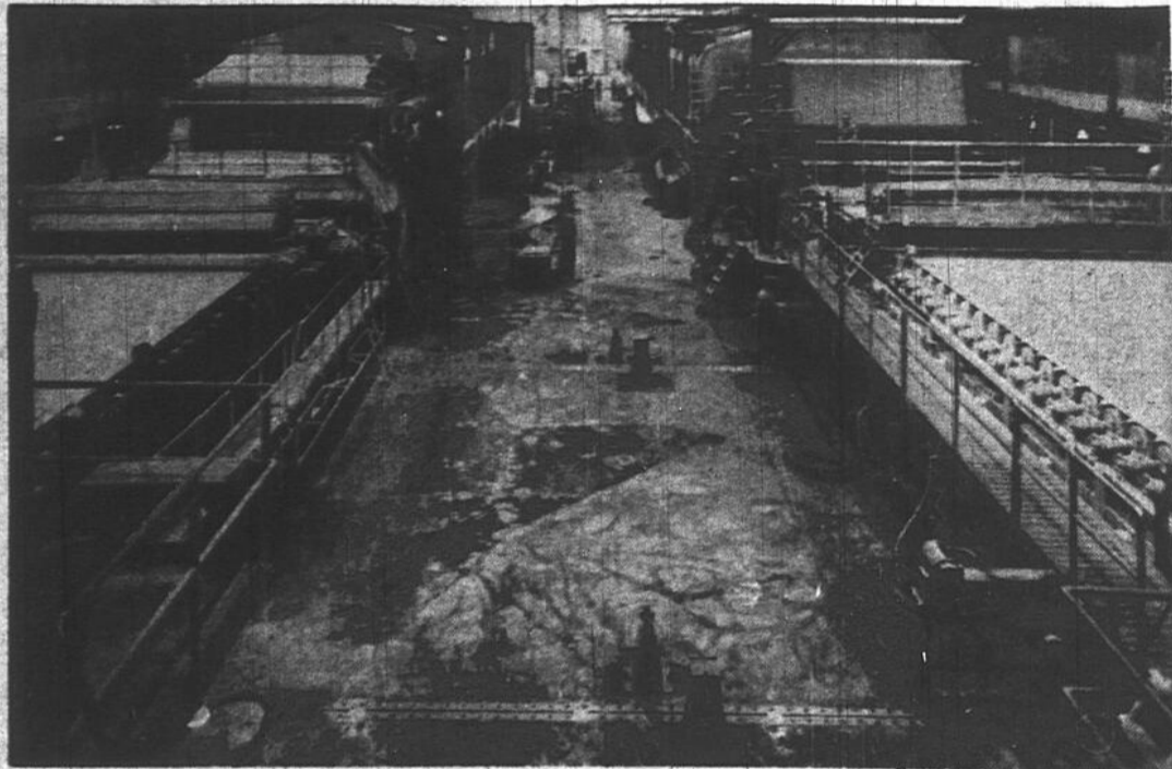
Les deux géants de la papeterie Rolland à côté l'un de l'autre : la nouvelle No 8 à droite, et la No 7 à gauche. Cette dernière a été mise en place en 1957.
