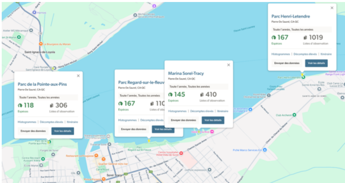
Voici les 4 sites publiques eBird, avec le nombre d'espèces pour chacun (en vert)
