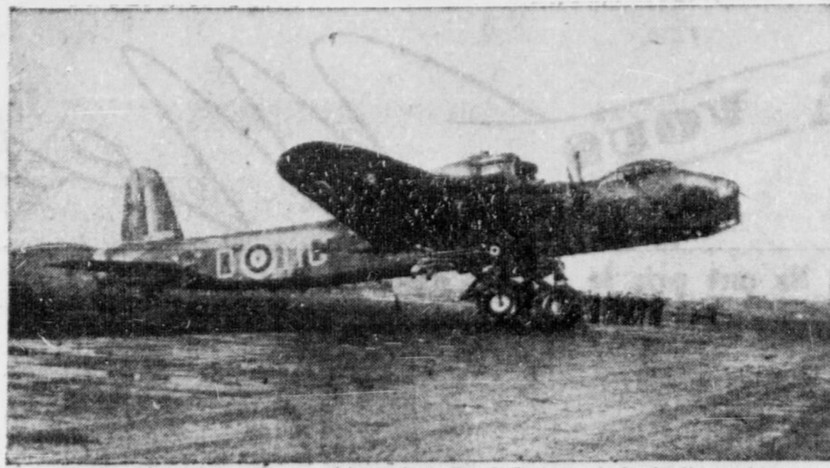
Une nouvelle addition à la puissance aérienne de la Grande-Bretagne: le bombardier quadrimoteur Short "Stirling". Il est propulsé par des moteurs en étoile de 14 cylindres Bristol "Hercules" ou Wright "Cyclone". D'une envergure de 90 pieds, il mesure 87 pieds 9 pouces de long et porte un formidable armement défensif. Train d'atterrissage et roue de queue sont escamotables.
