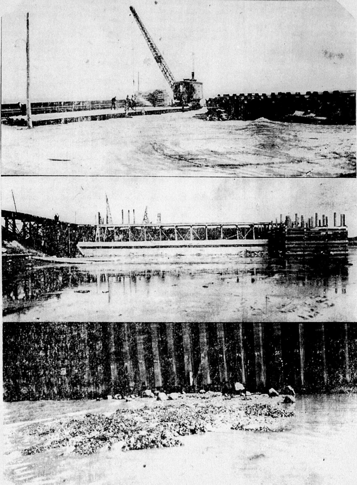
En haut, grue sur le vieux quai en train de manoeuvrer les paleplanches d'acier. Au milieu, charpente en bois. En bas, base des pilotis d'acier. Les morceaux de rocs épars donnent une idée des difficultés qu'on a rencontrées.
