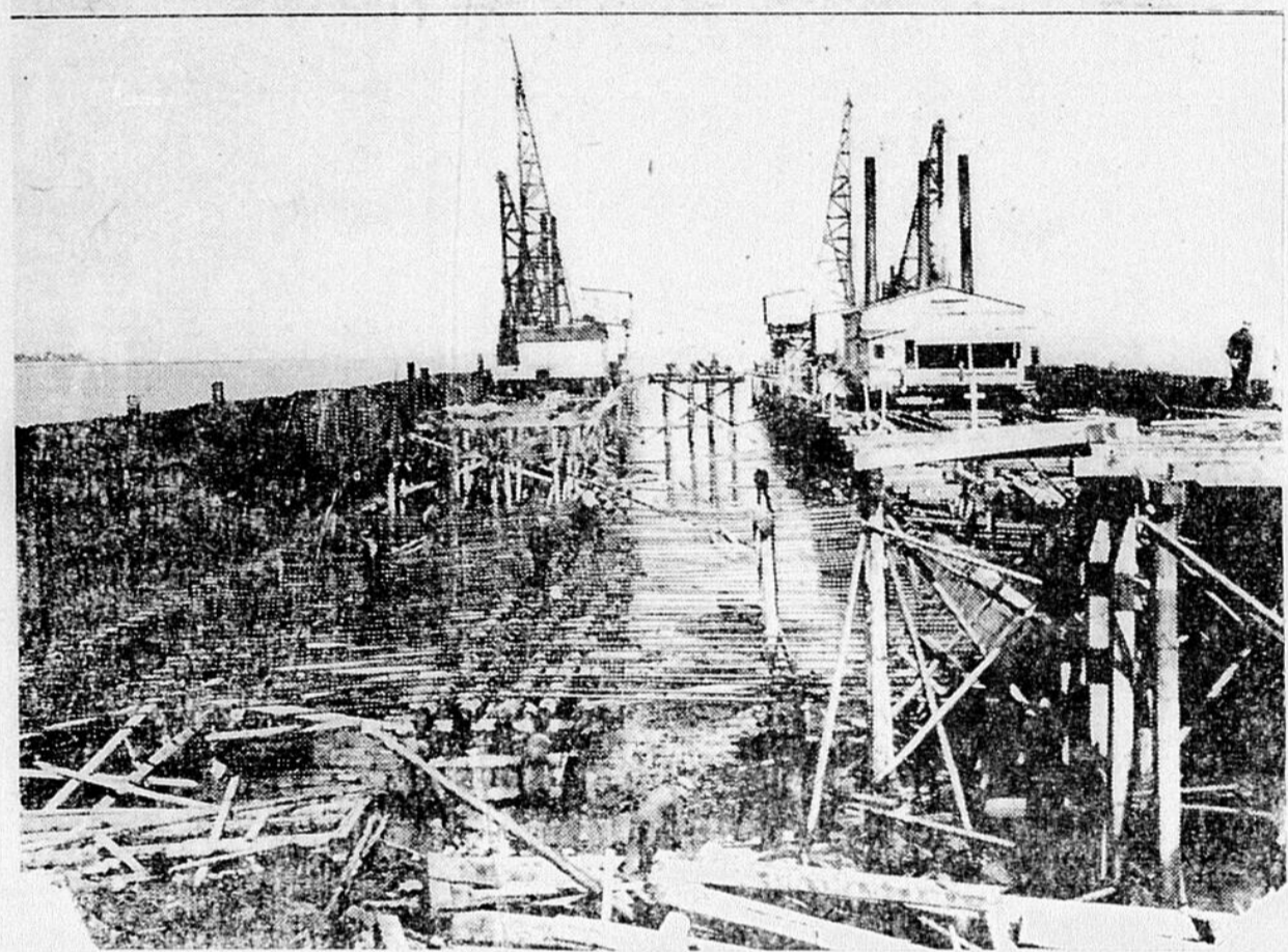
En haut, vue prise du vieux quai. On aperçoit les 4 grues qui acquièrent les ces pilotis ou paleplanche d'acier. En bas, état actuel des travaux. Cet
