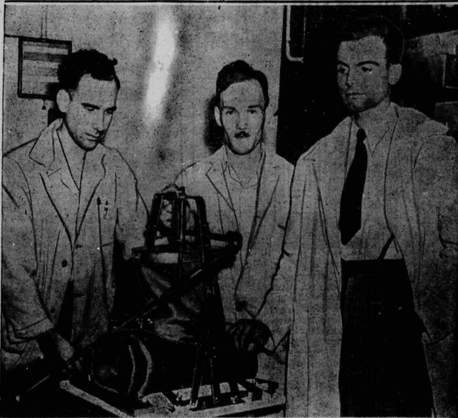
• Un nouveau genre de "respirateur" pour le traitement de la paralysie infantile des poumons a été inventé par Bernard Leybel, étudiant de 22 ans à l'Institut Banting à Toronto. Il diffère du respirateur Drinker ou "poumon de fer" dans lequel on enferme complètement le patient. La machine de Leybel construite en cuivre, se place tout contre l'abdomen du patient des hanches jusqu'au bas-estomac. Dans le haut il y a un diaphragme artificiel qui s'attache au bas de l'abdomen par un linge caoutchouté. Un moteur avec essieu et roue d'engrenage permet le mouvement du diaphragme de haut en bas, suivant le mouvement régulier de la respiration. Il donne les mouvements d'expansion et de contraction à l'estomac comme dans la respiration naturelle. Bernard Leybel (à droite) regarde son invention avec ses techniciens Leonard Brock, à gauche, et Jack Conley, au centre.
