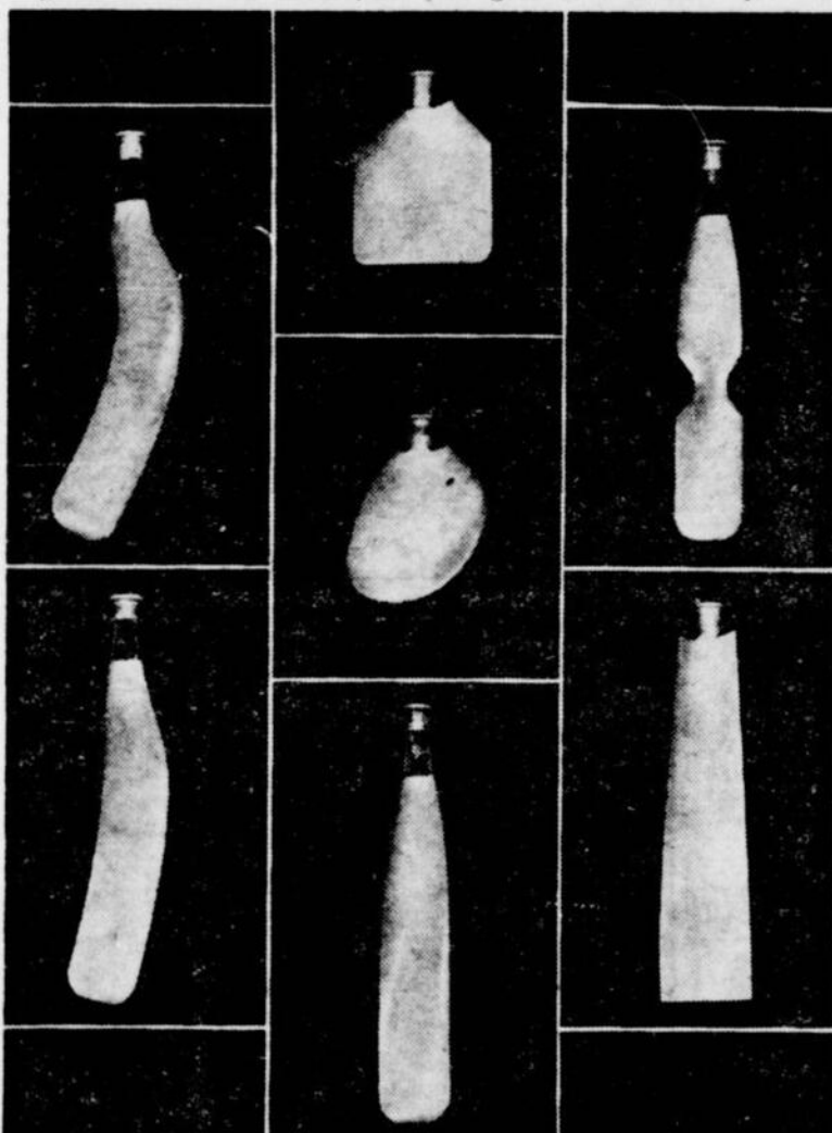
Voici quelques-unes des formes de pales qui ont été mises à l'essai pour servir aux moteurs à réaction. Celle du haut, à gauche, a été choisie. Elle permet à l'hélice d'atteindre un rendement de 80 p.c. à 600 milles à l'heure.
