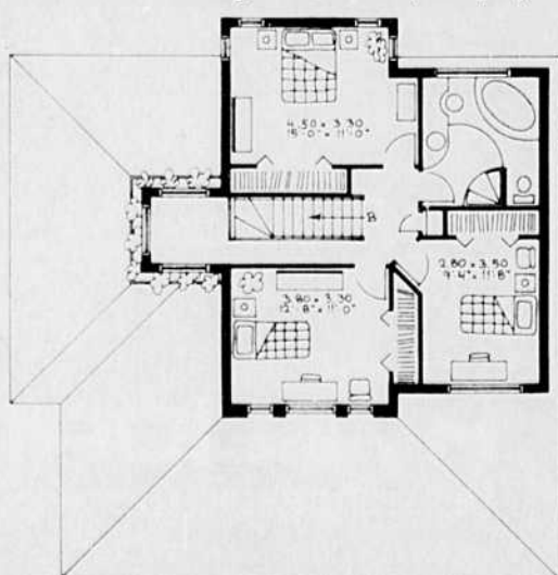
Étage: 72,18 m 2 (802 pi 2 )
