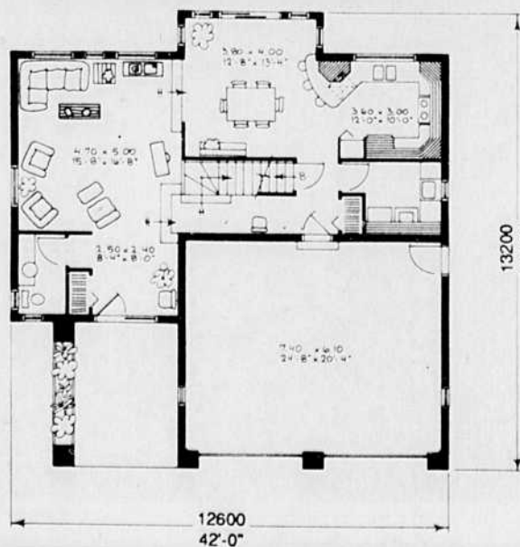
Rez-de-chaussée: 84,6 m 2 (940 pi 2 )
