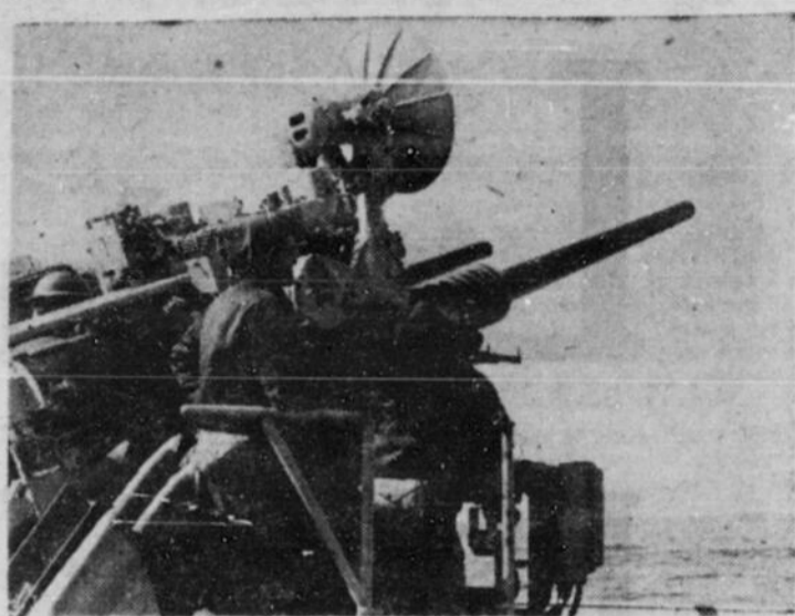
A L'ACTION. — L'"Haida" était le seul destroyer canadien actif au large de la Corée le 2 juin dernier. Pour marquer l'avènement de la Reine, il a détruit deux trains de ravitaillement. On voit dans la photo ci-dessus des marins de l'"Haida" qui se tiennent en attente près d'un canon de trois pouces. En avant, on remarque le matelot Kenneth Brown, de Belmont (N.-E.). (Photo de la Défense nationale)
