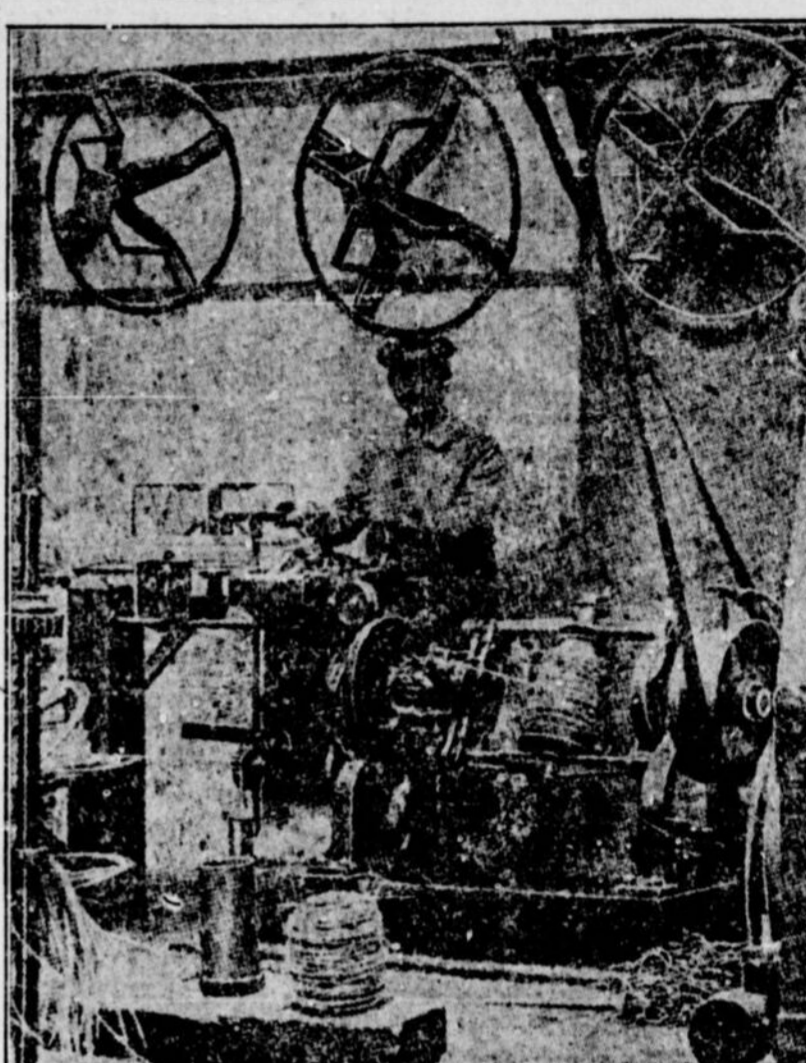
MACHINE A FABRIQUER LA RONCE ARTIFICIELLE
