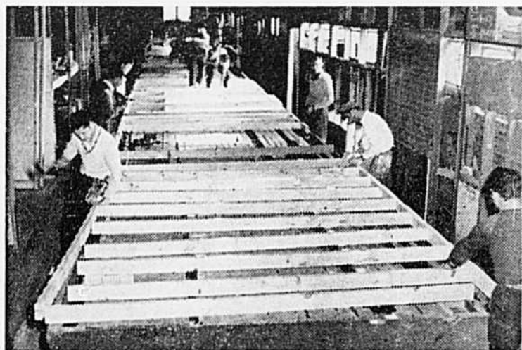
Les murs sont fabriqués sur une chaîne d'assemblage, à plat.
