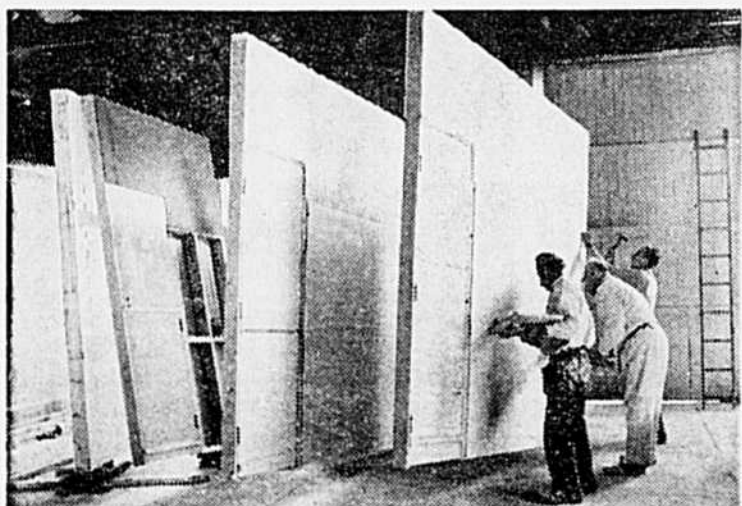
Les murs redressés, les ouvriers posent les portes, les fenêtres, etc.
