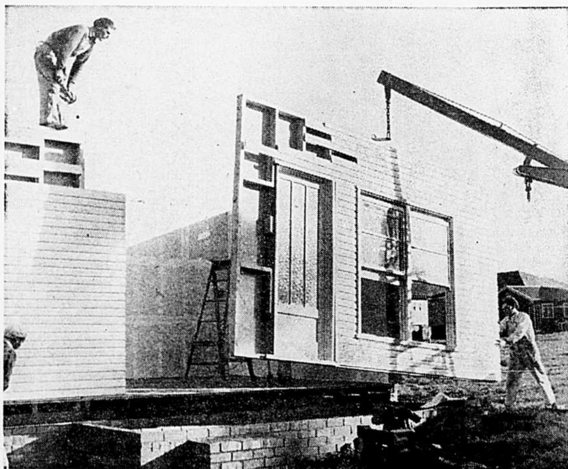
Comme un jouet, le mur est soulevé à l'aide d'une grue et posé sur les fondations.
