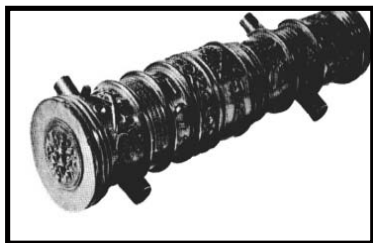
Canon de siège allemand (début du XVI e siècle)
