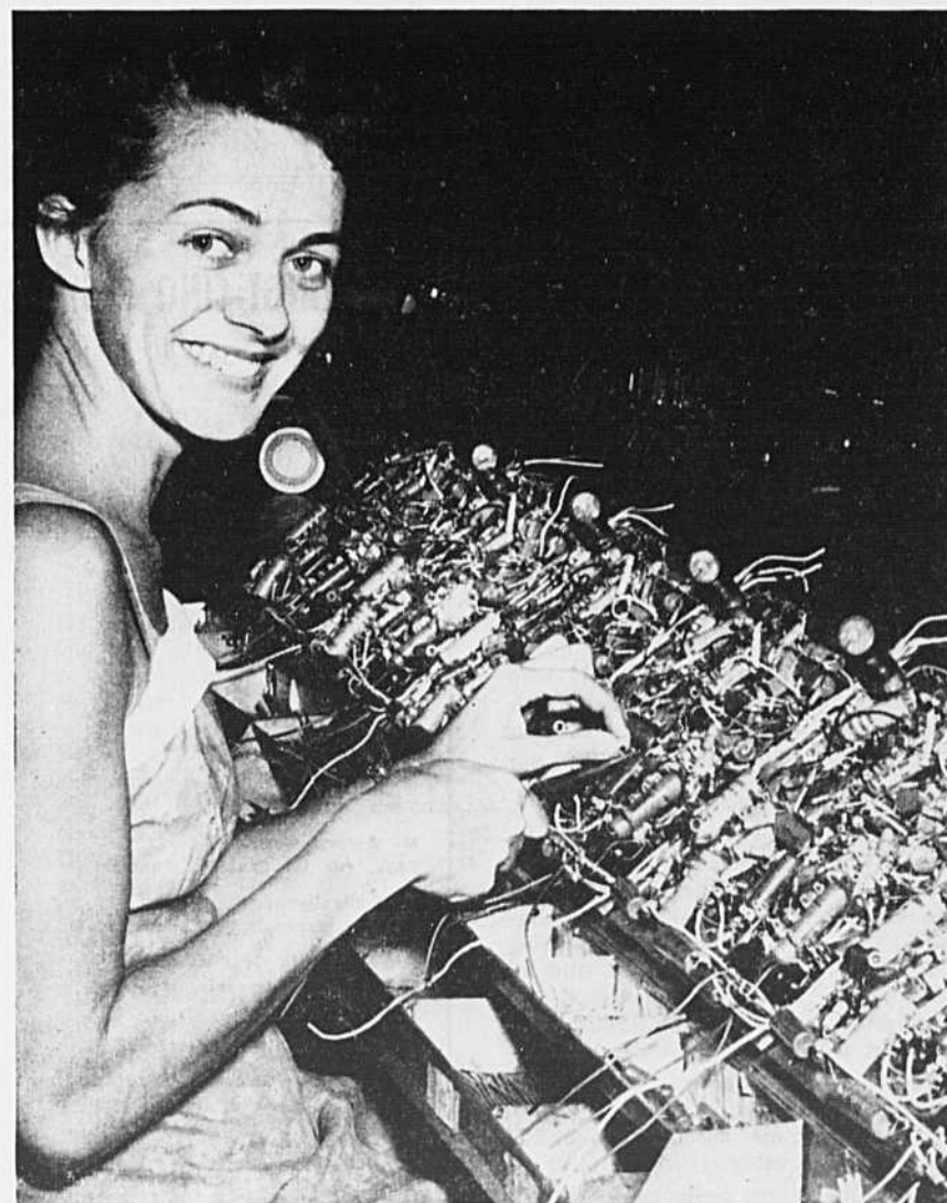
1,400 PIÈCES ET PLUS. — Vous avez là, sous les yeux, l'intérieur d'un appareil de télévision Canadian Westinghouse. Dans un poste récepteur de ce genre on compte 1,400 pièces au moins. L'assemblage et la mise en place de ces pièces multiples exige une très grande dextérité et de la compétence.
