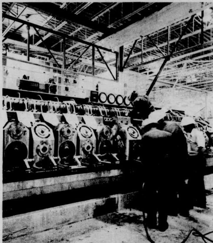
A la nouvelle usine de fil machine d'Arvida, les cages du laminoir sont interchangeable, sauf pour la première cage et pour les rouleaux de travail. Ainsi, une cage peut-être remplacée en cinq minutes assurant un régime de production élevé et régulier.
