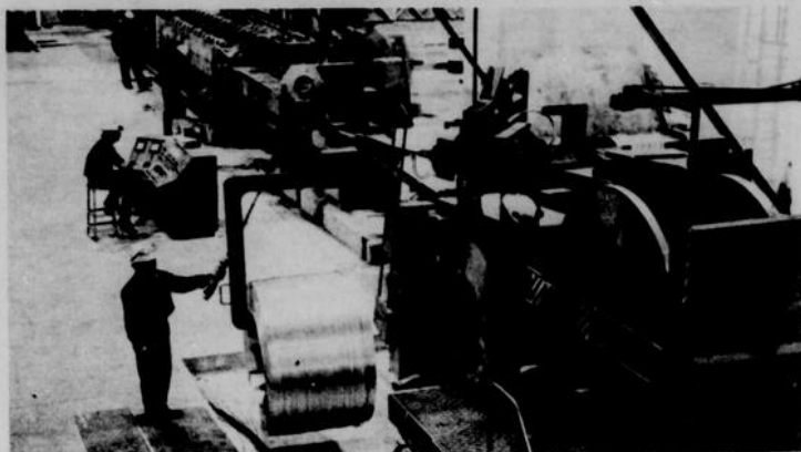
L'aluminium en fusion est analysé, allié, puis versé dans une grande roue de coulée. Il sort sous forme de barres de 5.2 po. car, de section qui passe ensuite dans un appareil de trempe avant d'être entraîné à travers 15 cages de laminoir. Les rouleaux de ce laminoir sont disposés à 120° l'un de l'autre et la barre d'aluminium y est transformée en fil machine de 3/8 de po. de diamètre.
