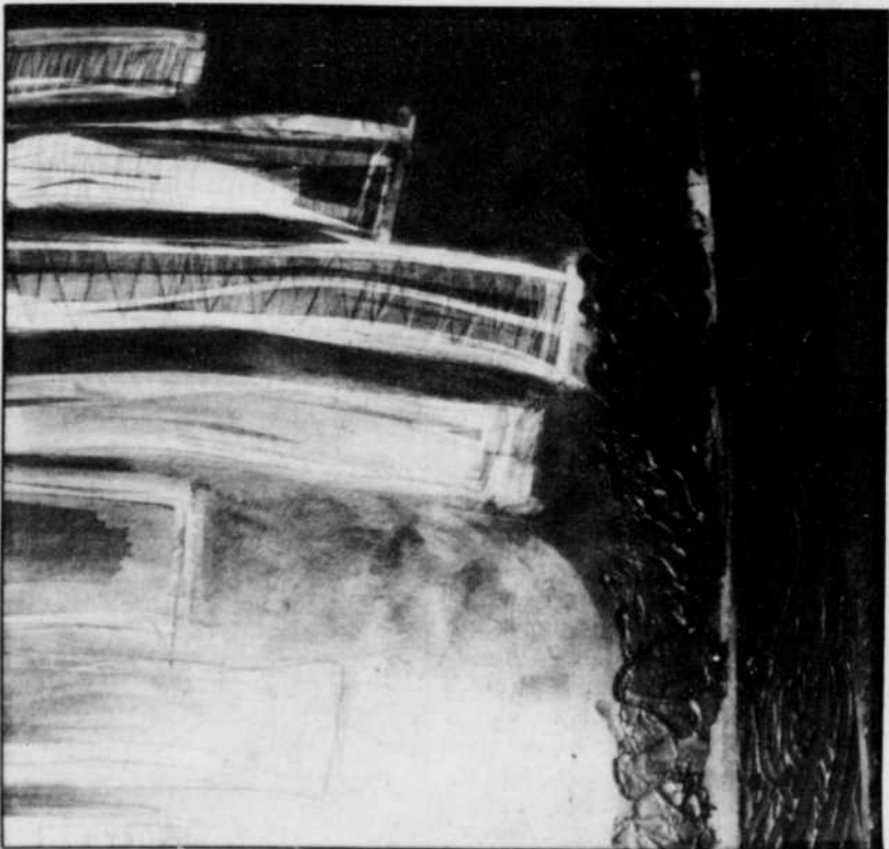
Sur fond sombre, les bandes d'énergie de Guylaine Doucet
