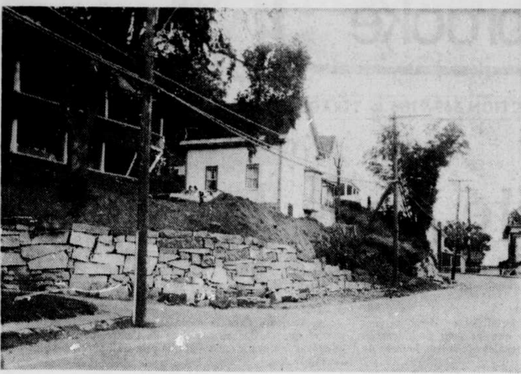
Les employés de la ville de Rock Island ont plus de la moitié du travail d'effectué à la réparation du mur de soutènement de la rue Railroad. Ce mur à la suite de la venue du printemps menaçait de s'écrouler. Les autorités de la ville économiseront quelques milliers de dollars en faisant faire ces travaux par leurs employés qui semblent être experts dans la matière.
